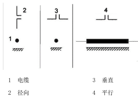
图 B.3 地面敷设法中的天线方向
